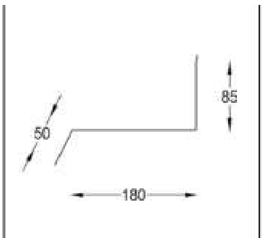
SCOSSALINA DI RACCORDO FUSTELLATA FIG. 3
