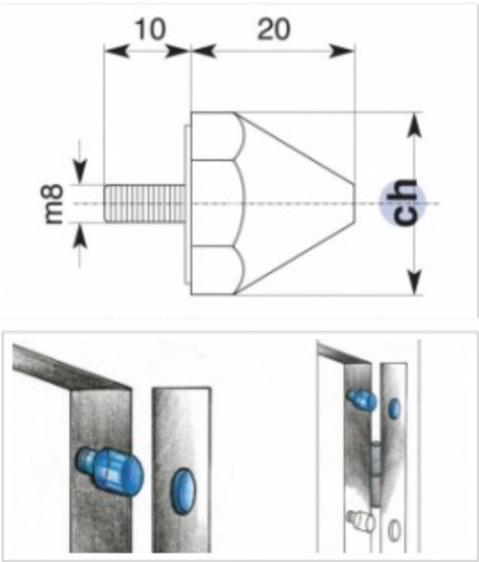
Art. 445/EG-445/E Antistrappo per porte blindate
